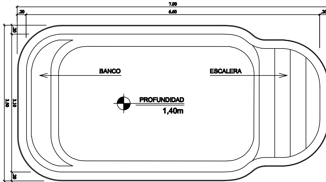
DIBUJO TÉCNICO
