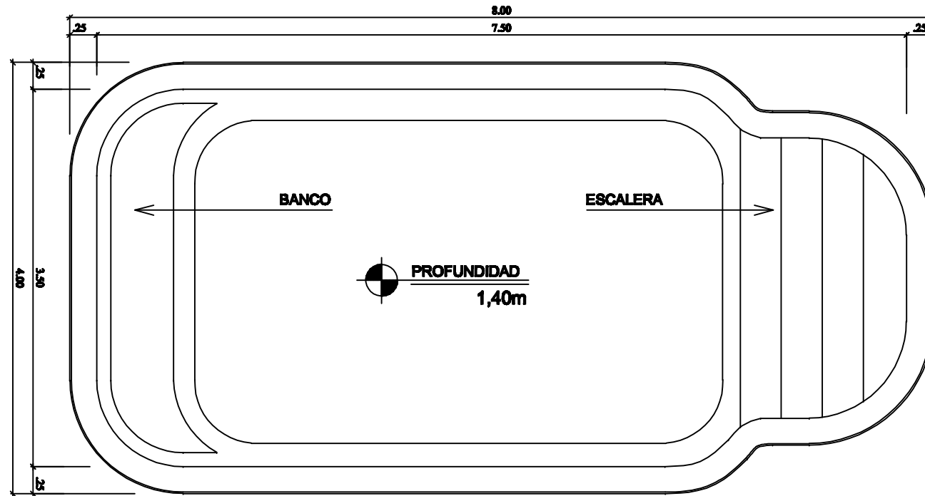
DIBUJO TÉCNICO ESCALA 1:50
