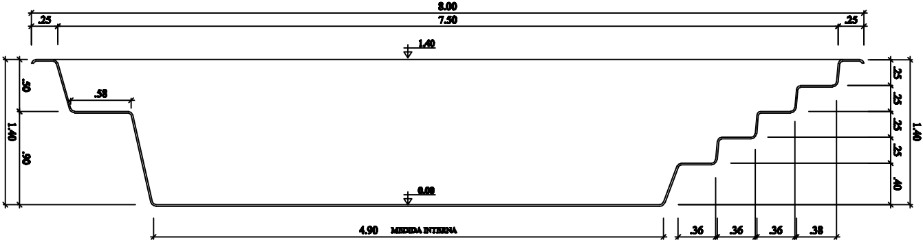
CORTE LONGITUDINAL ESCALA 1:50
