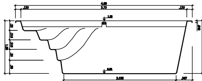
CORTE LONGITUDINAL ESCALA 1:20
