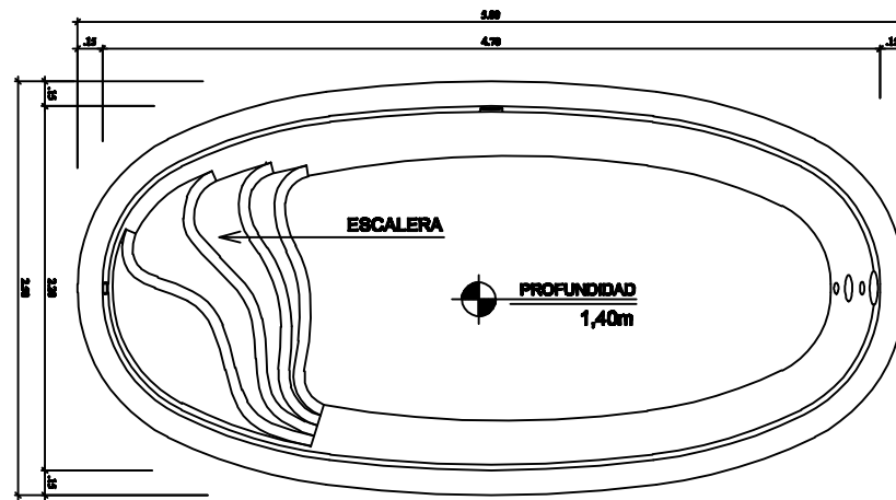
DIBUJO TÉCNICO ESCALA 1:50
