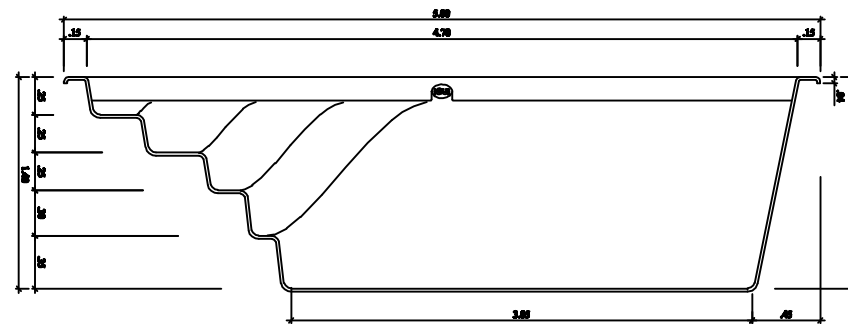
CORTE LONGITUDINAL ESCALA 1:50
