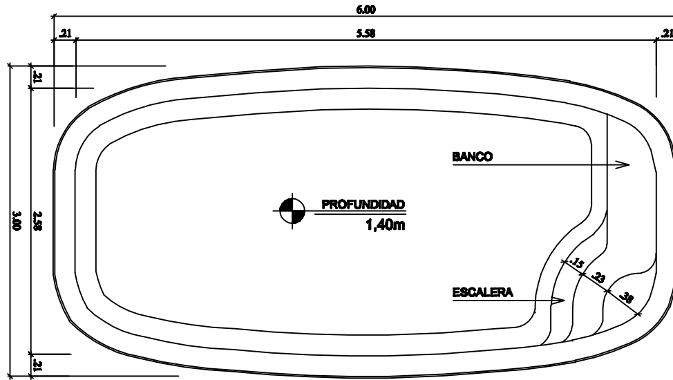
DIBUJO TÉCNICO ESCALA 1:50
