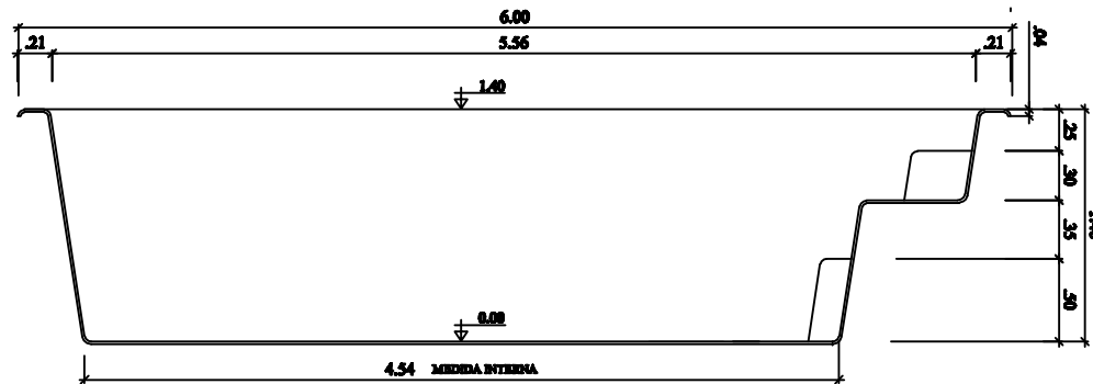
CORTE LONGITUDINAL ESCALA 1:50
