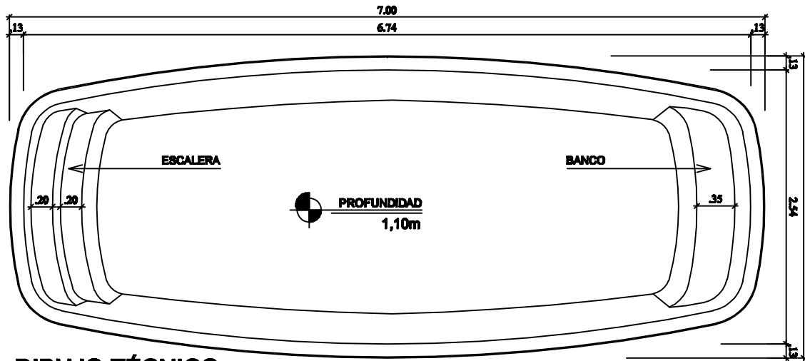
DIBUJO TÉCNICO ESCALA 1:50
