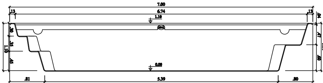
CORTE LONGITUDINAL ESCALA 1:50
