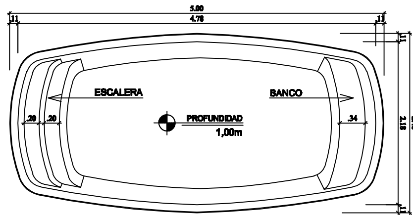
DIBUJO TÉCNICO ESCALA 1:50
