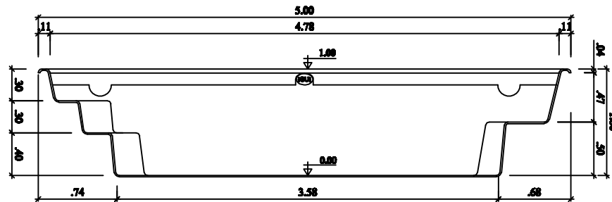
CORTE LONGITUDINAL ESCALA 1:50
