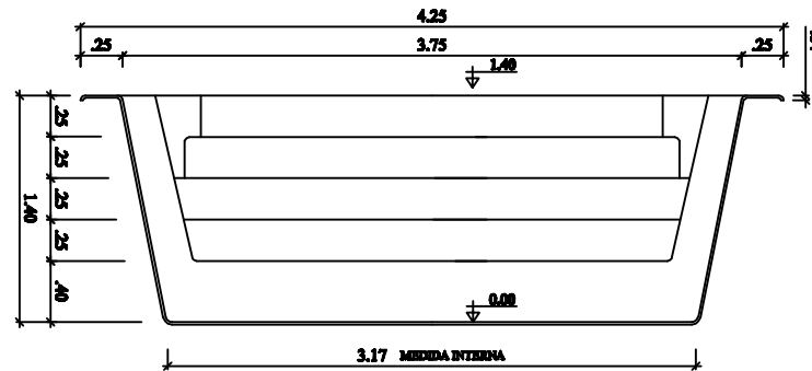
CORTE TRANSVERSAL ESCALA 1:50
