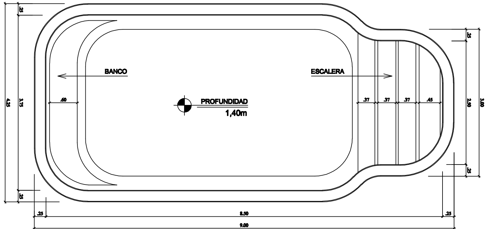
DIBUJO TÉCNICO ESCALA 1:50
