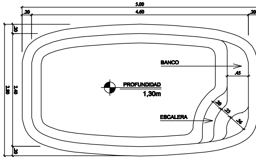
DIBUJO TÉCNICO ESCALA 1:50
