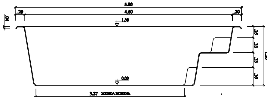
CORTE LONGITUDINAL ESCALA 1:50
