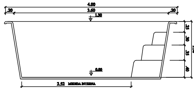
CORTE LONGITUDINAL ESCALA 1:50
