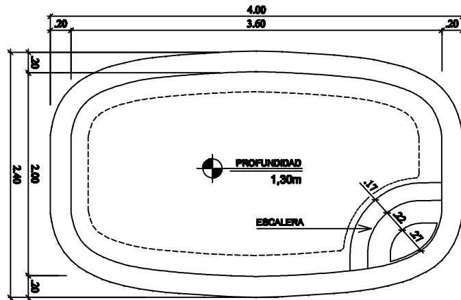
DIBUJO TÉCNICO ESCALA 1:50
